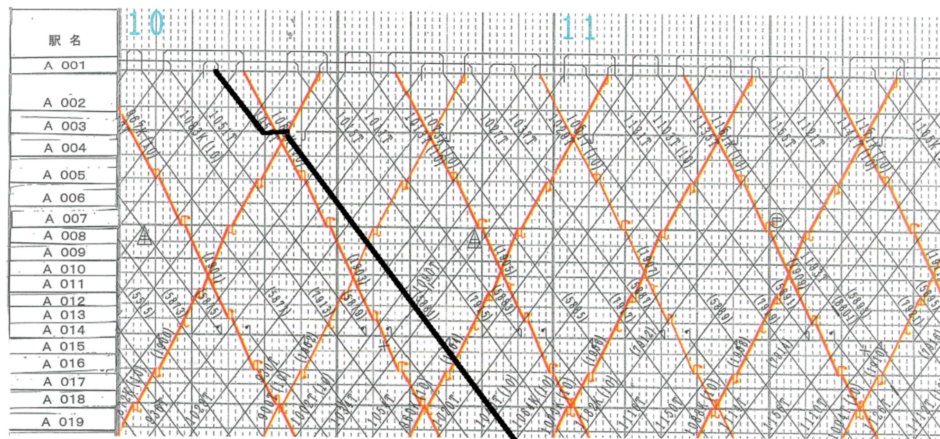
図4 ダイヤグラム（列車運行図表）
